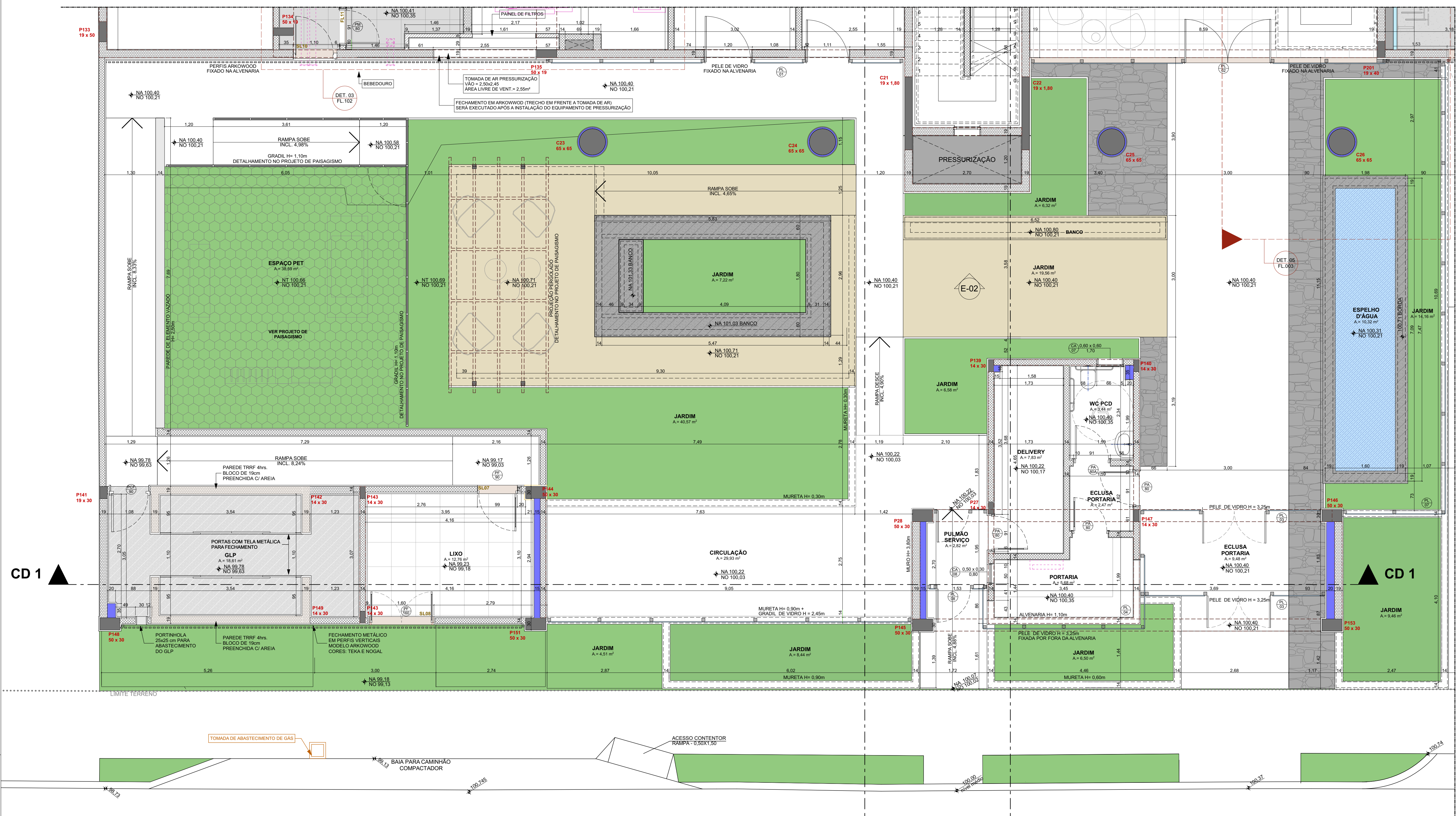
DETALHE ENTRADA TÉRREO PORTARIA E ÁREAS DE CONVÍVIO EXTERNA ESC.:1:50
