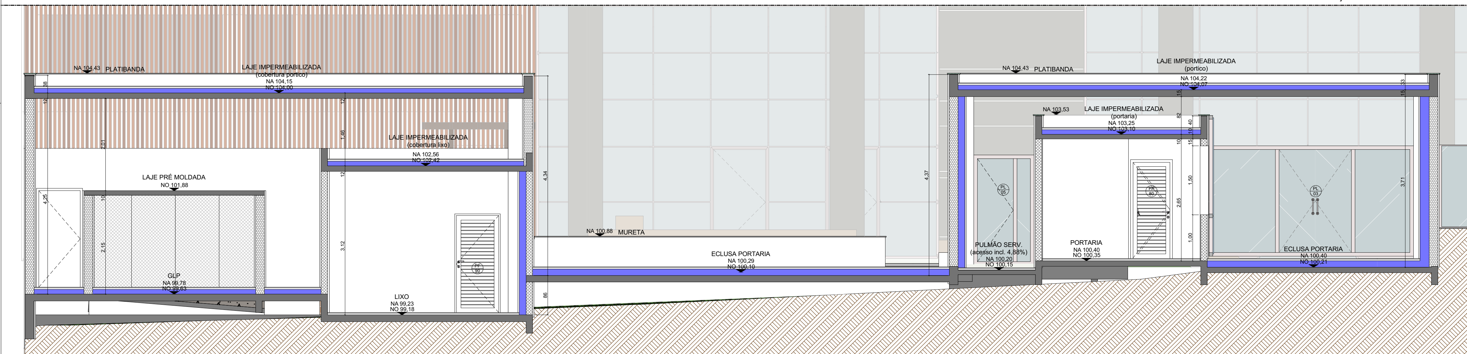
CD 1 CORTE ESC.:1:50
