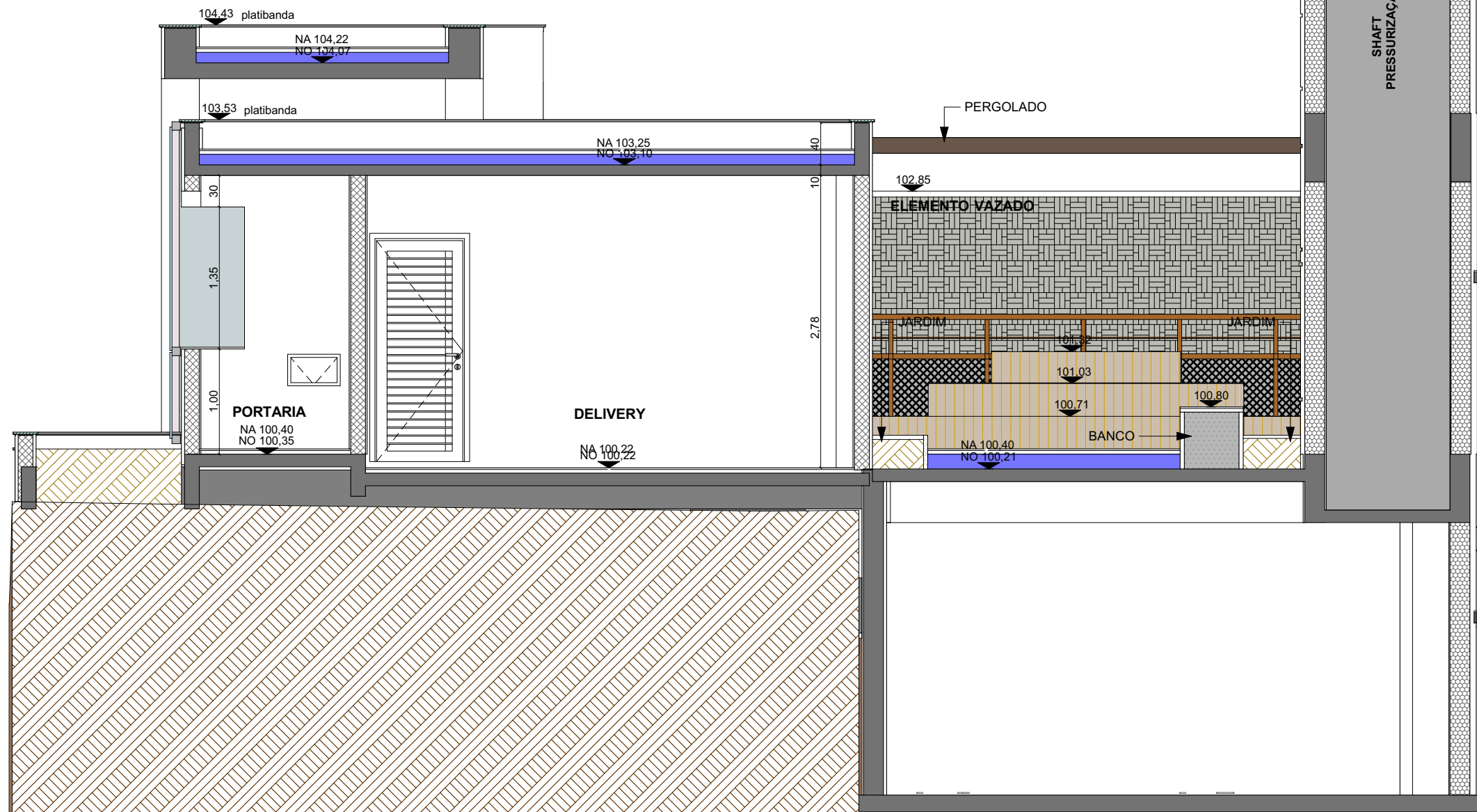
B CORTE ESC.:1:50
