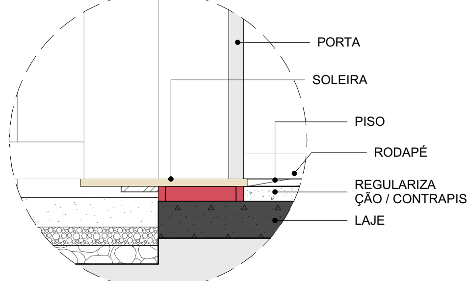
DETALHE SOLEIRA
