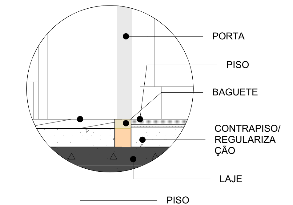
DETALHE BAGUETE
