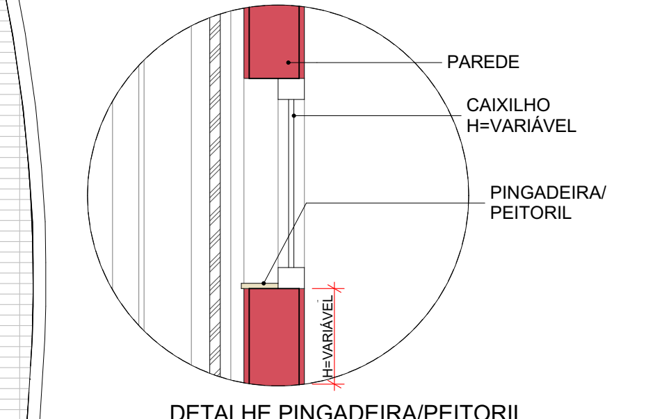
DETALHE PINGADEIRA/PEITORIL
