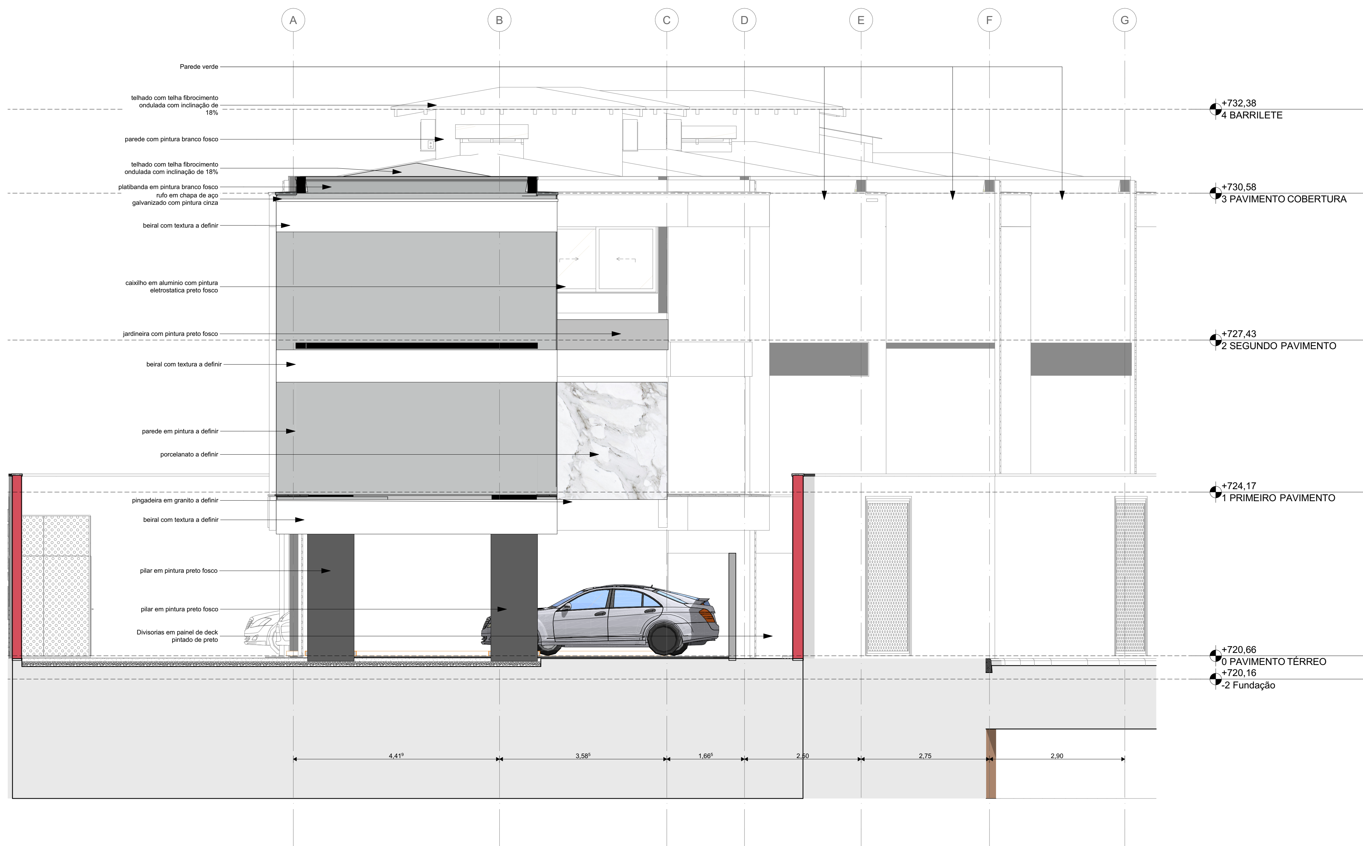
2 Elevação Escala: 1:50
