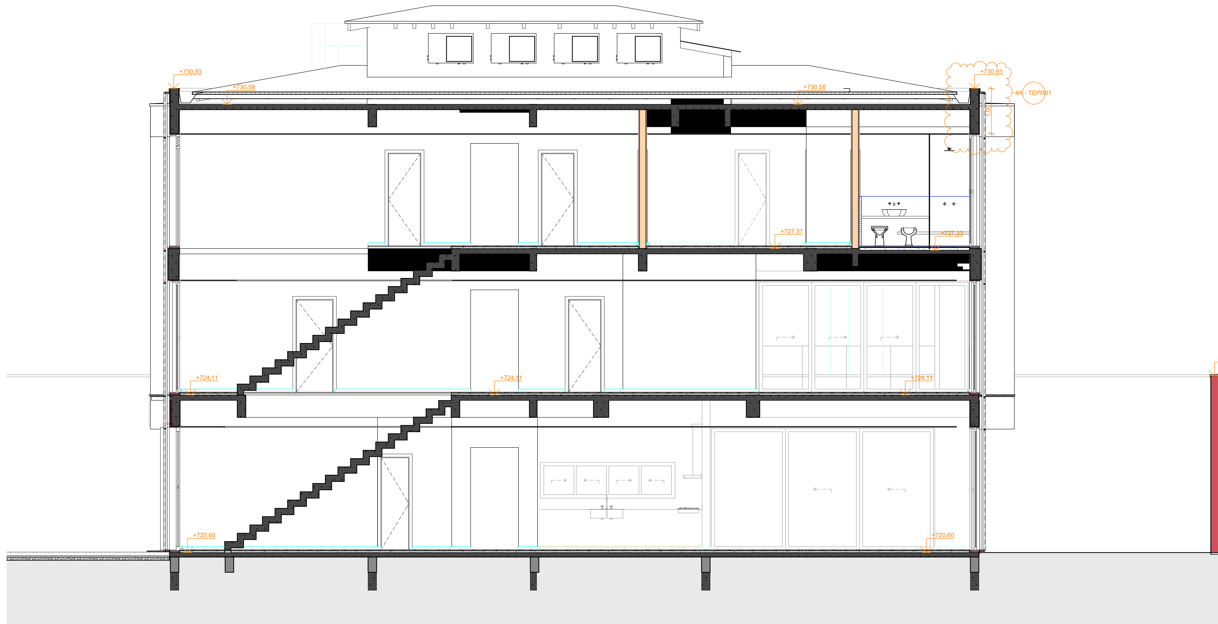
BB Corte Escala: 1:50
