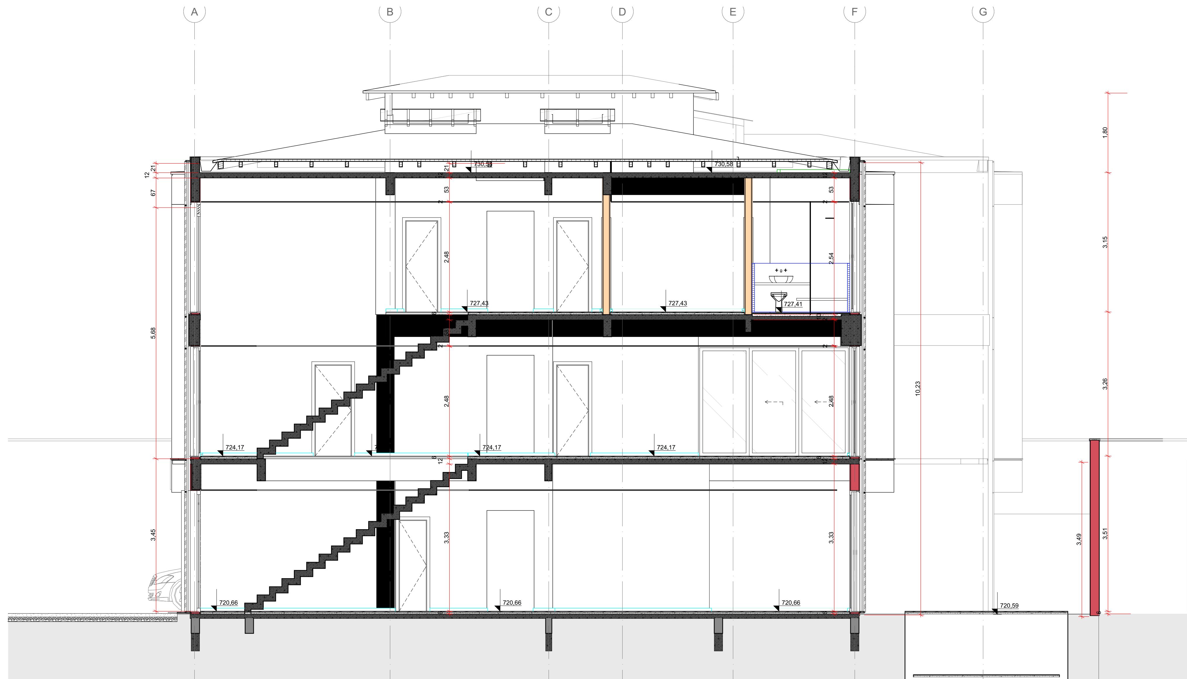
DD Corte Escala: 1:50
