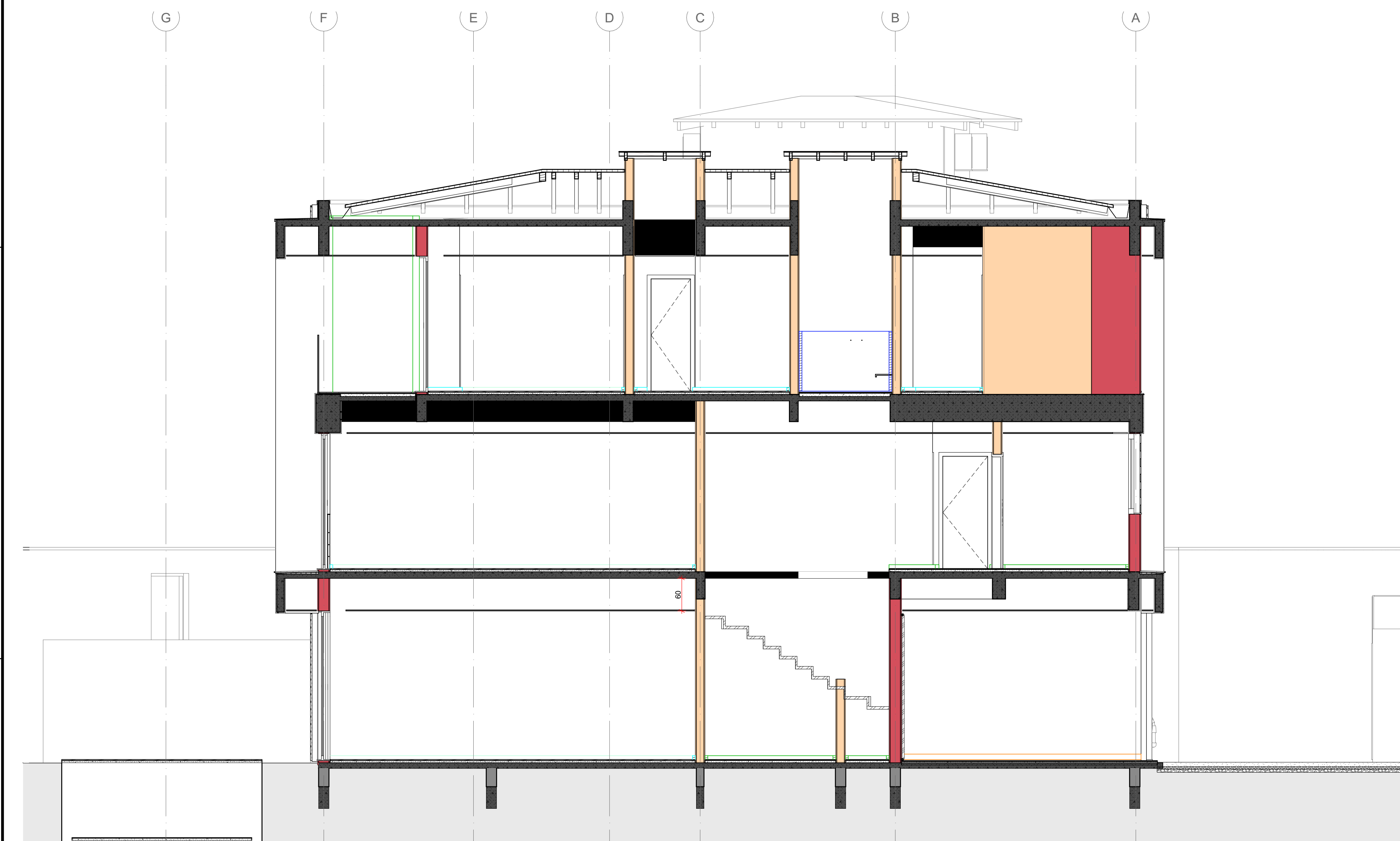
CC Corte Escala: 1:50
