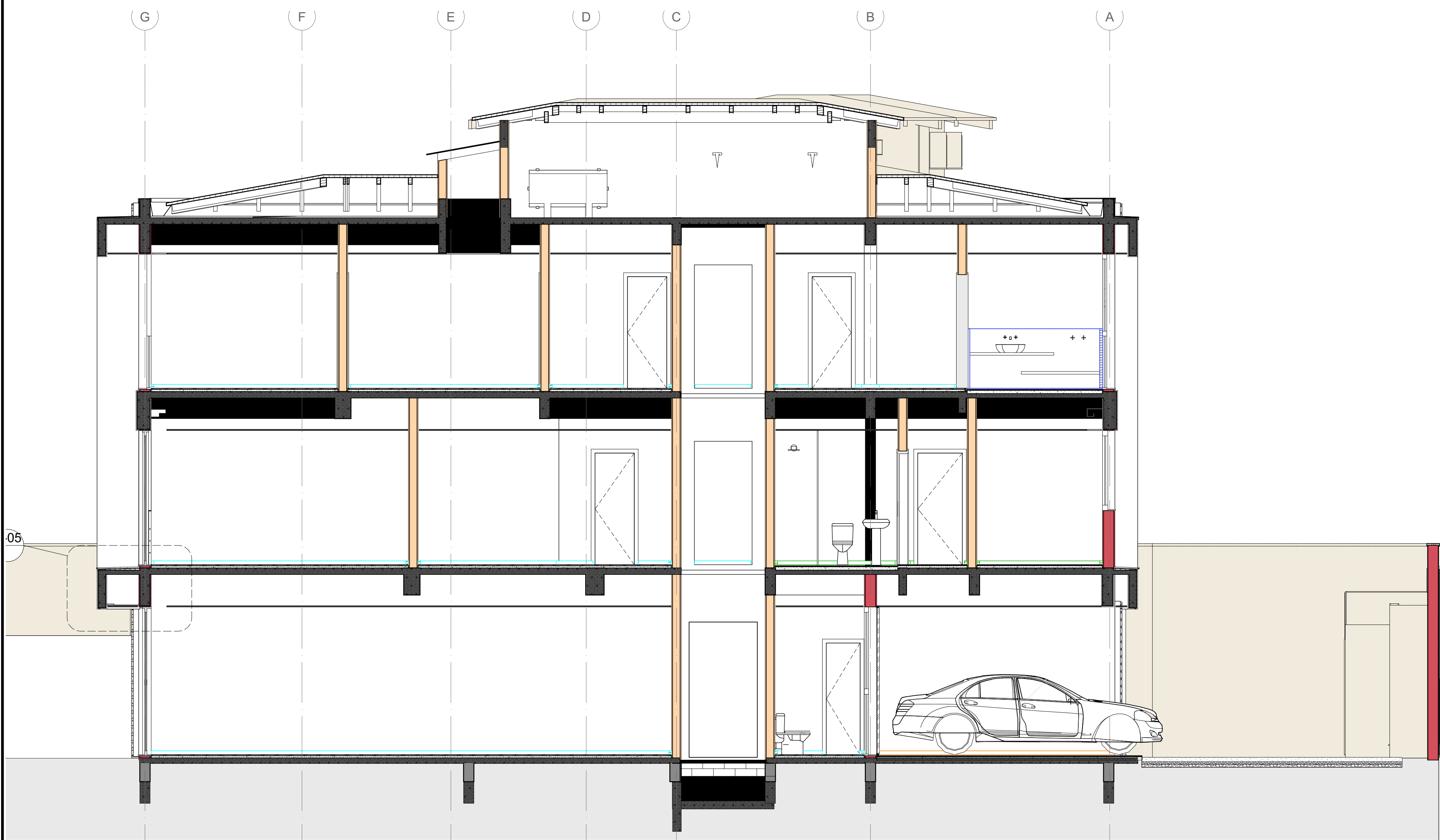
AA Corte Escala: 1:50
