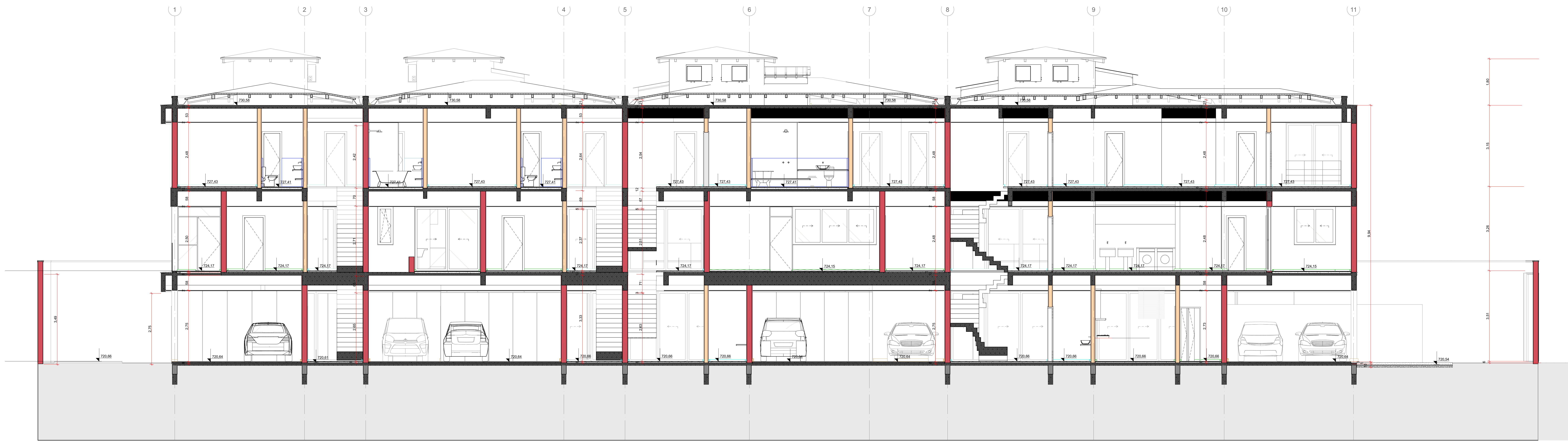
II Corte Escala: 1:50
